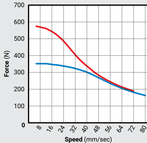
NEMA23 • 10 x 8 mm
